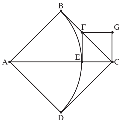
FIG. 1 - L'anthyphèrese de la diagonale et du coté du carré
