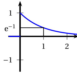
Figure 1 : représentation de la fonction s_1
